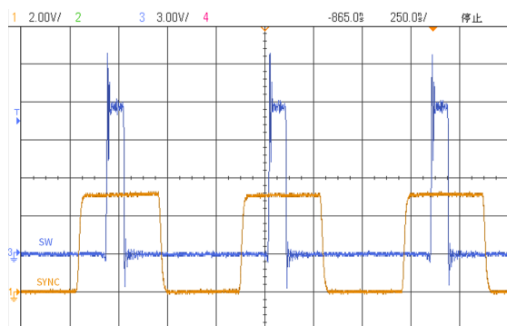
图 13-7 SYNC=1200KHz Plot
