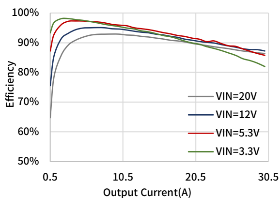
图 13-2 Efficiency 1.2V Output
