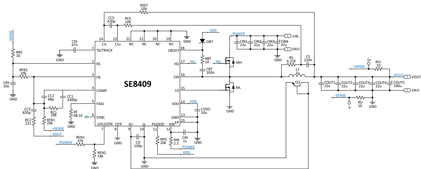
图 4 SE8409 典型应用拓扑 VIN=12V, VO=1.2A, IO=25A
