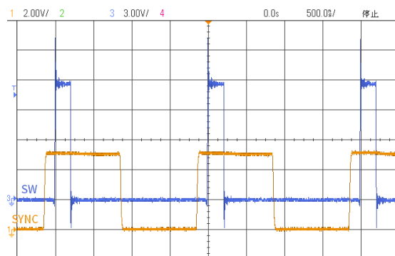
图 13-8 SYNC=500KHz Plot
